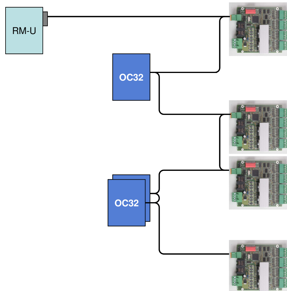
Fig. 13 : Câblage réseau entre les modules Dinamo, exemple de méthode 1
