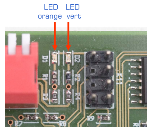
Fig. 16 : TM44 LED
