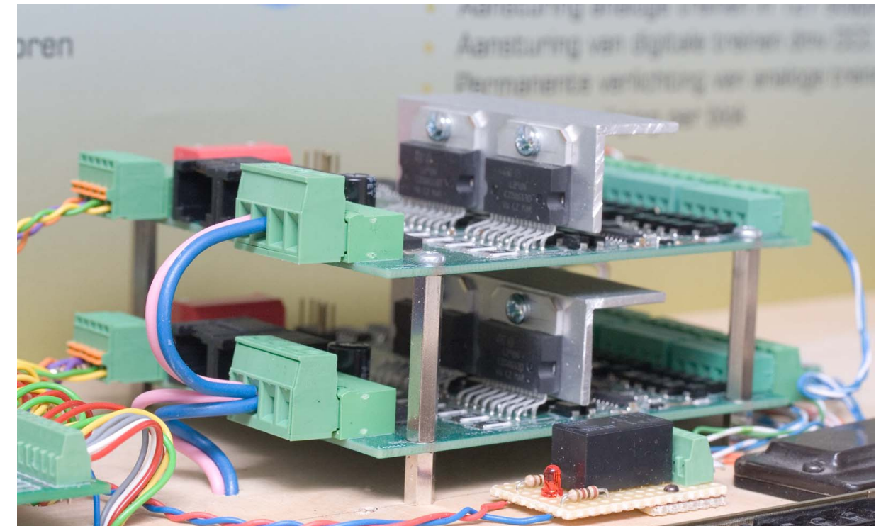
Fig. 3 : Montage de plusieurs TM44
