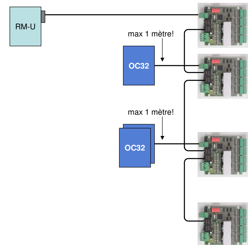
Fig. 14 : Câblage réseau entre modules Dinamo, exemple de méthode 2
